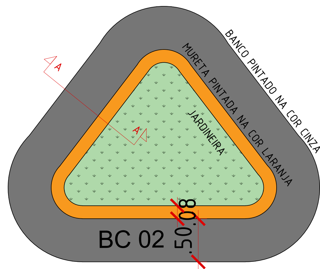
DETALHE BANCO BC 02 PLANTA BAIXA ESC-1/50
