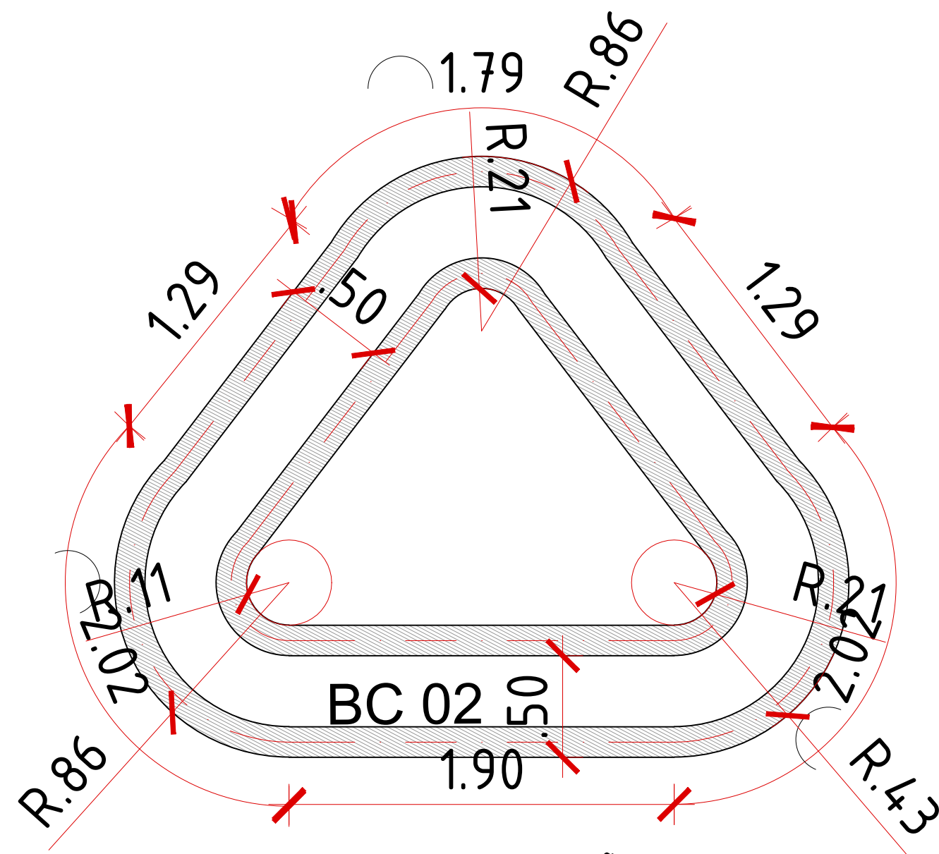
COMPOSIÇÃO DAS ALVENARIAS PLANTA BAIXA ESC-1/50
