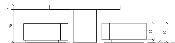
DETALHE MESA VISTA ESC-1/25
