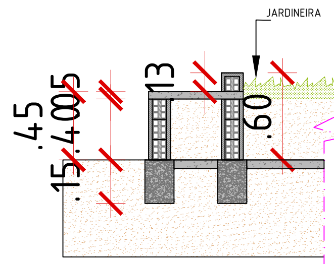
CORTE "A-A" BANCO BC-02 PLANTA BAIXA ESC-1/50
